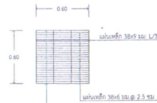
ขยายฝาเหล็ก มาตราส่วน No Scale
