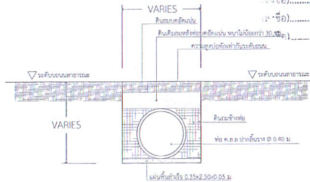
รูปตัด B มาตราส่วน No Scale
