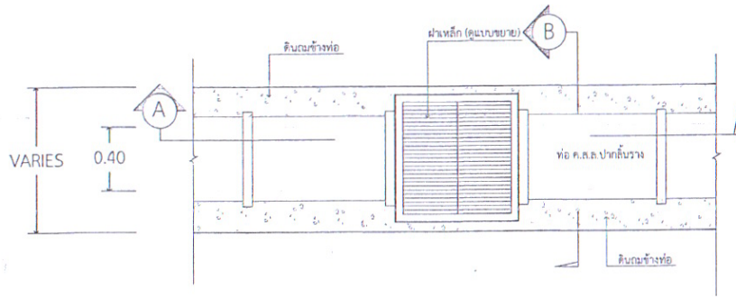
แปลนบ่อพักและท่อ ค.ส.ล. 0.40 ม. มาตราส่วน No Scale
