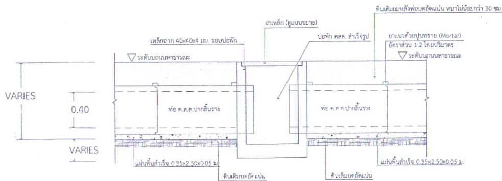
รูปตัด A มาตราส่วน No Scale
