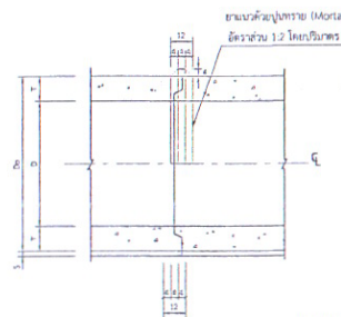
แสดงรูปตัดท่อ ค.ส.ล. มาตราส่วน No Scale
